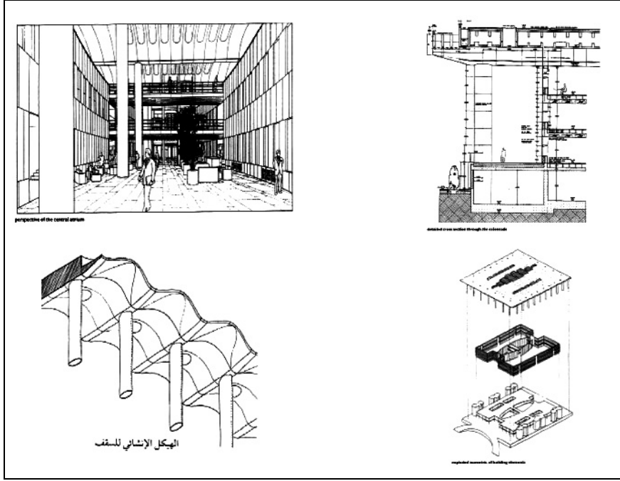
شكل رقم ٢١ - تسجيل الفكر الإنشائي للمشروع من واقع رسومات المصمم
